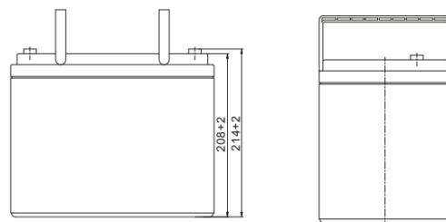
■ T6-A Terminal Unit: mm
