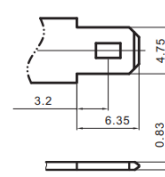
■ T1 Terminal
